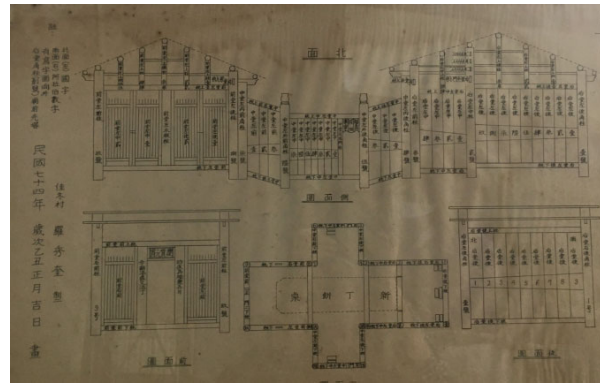
圖 9 羅秀奎福廠繪製圖(2)
